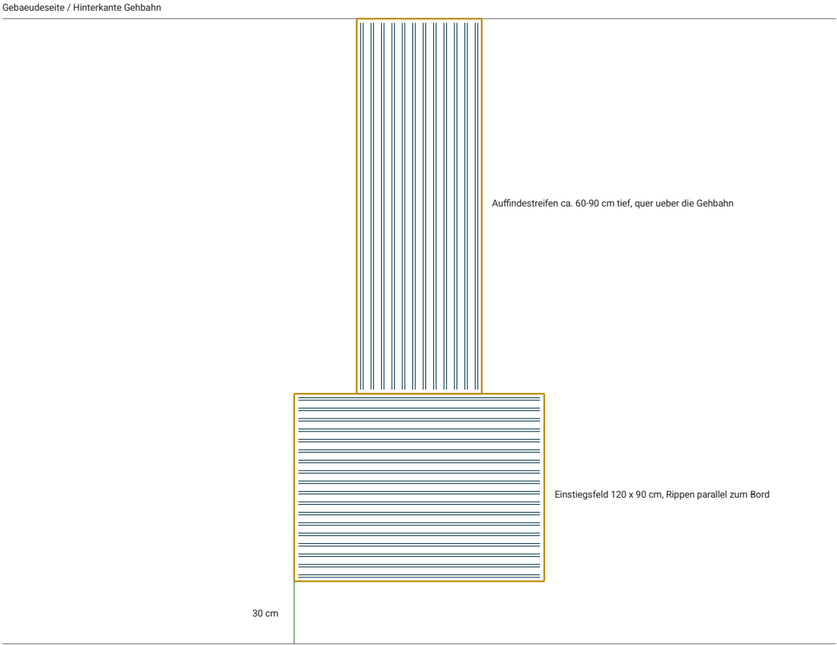
5 Bushaltestelle: Einstiegsfeld an der vorderen Tuer
