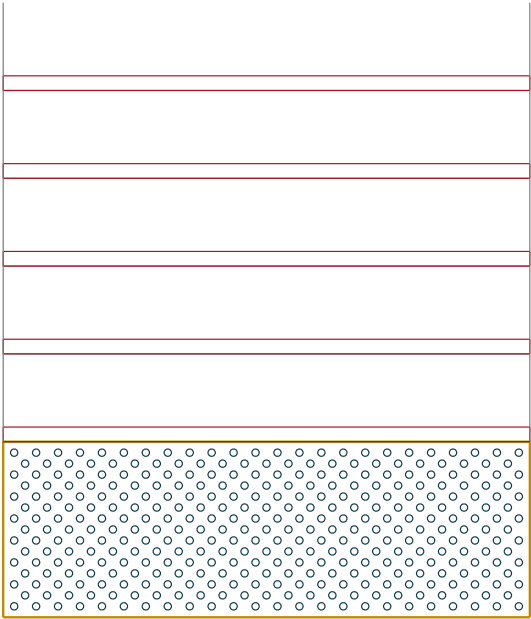
4 Aufmerksamkeitsfeld vor Treppe gesamte Treppenbreite, mind. 60 cm tief; Stufenkante 4-5 cm (DIN 18040-1)
